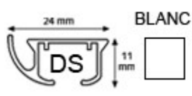
Rail DS Simple tout équipé sur mesure - 10 glisseurs par mètre - Embout avec arrêt à vis
